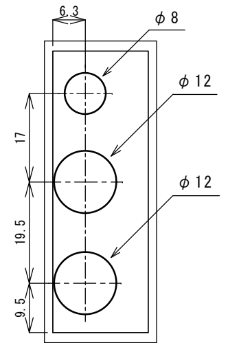
パネル加工図
