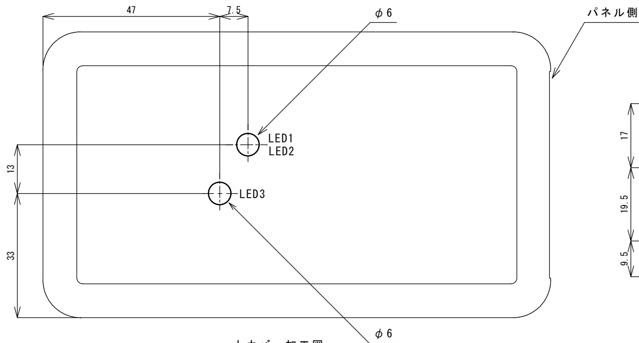
上カバー加工図
