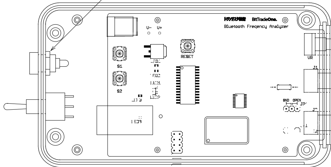
下カバー内側
